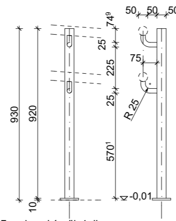
O7 oszlop - készül: 1 db m 1:20
