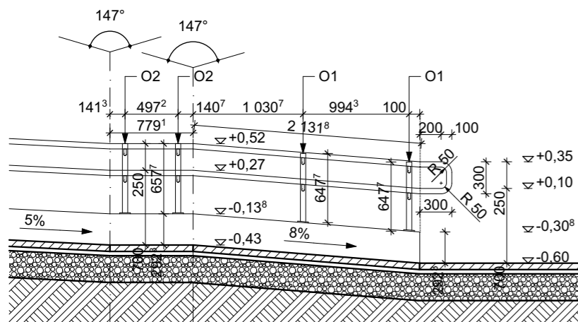
1. nézet m 1:50
