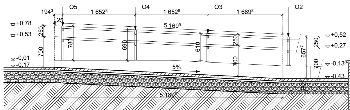
2. nézet m 1:50
