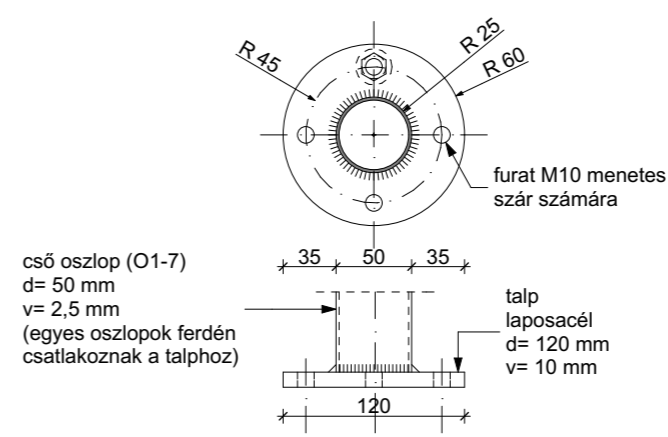
Oszlop talp - készül: 9 db m 1:5
